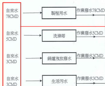
附件 12 用水及排水之平衡關係圖
